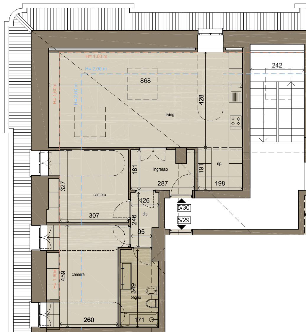
APPARTAMENTO 5/30 SCALA 1:100
