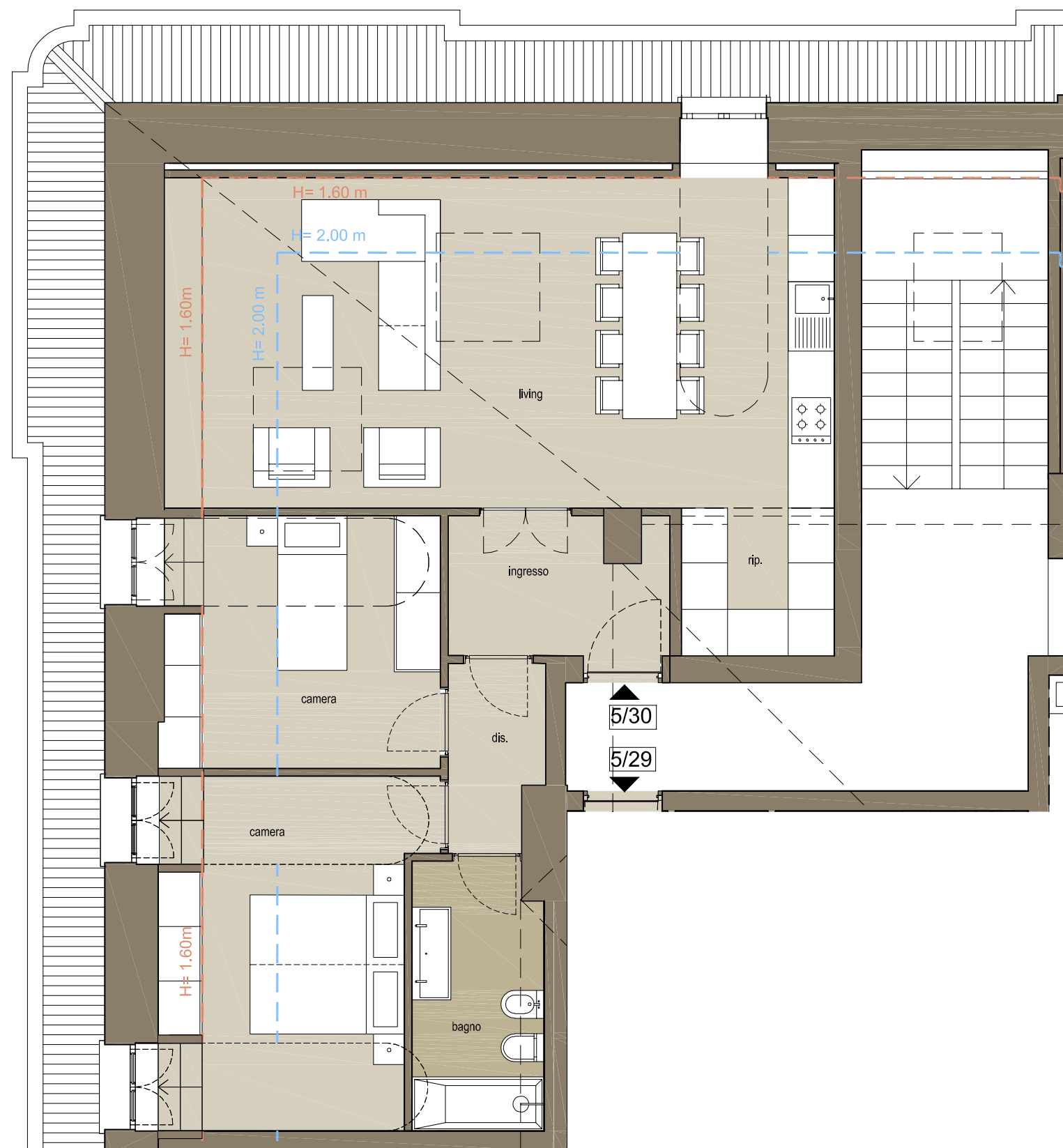
APPARTAMENTO 5/30 (FUORI SCALA)
